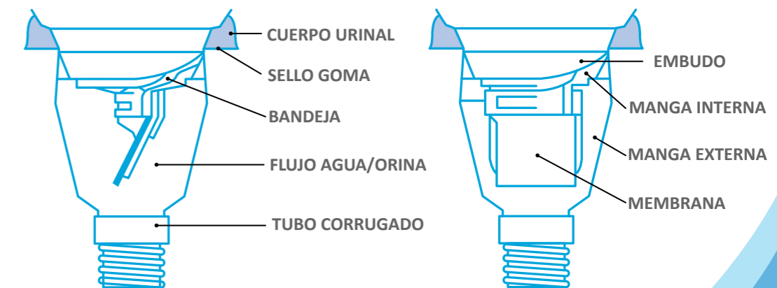
CORTE LATERAL - TRAMPA DE OLORES SECO
